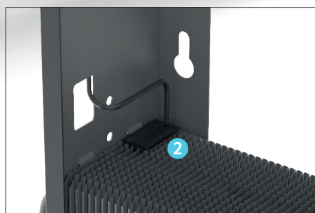
2 Klik de watertempatuursensor op de warmtewisselaar.
